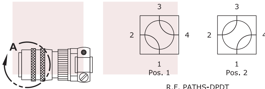
R.F. PATHS-DPDT
