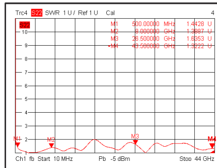
Output VSWR @+85°C
