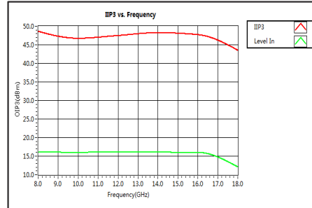
IIP3
