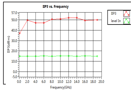
IIP3
