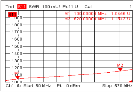
Input VSWR @+60°C
