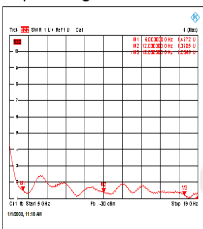
Output VSWR @+25°C
