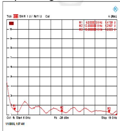
Output VSWR @-40°C
