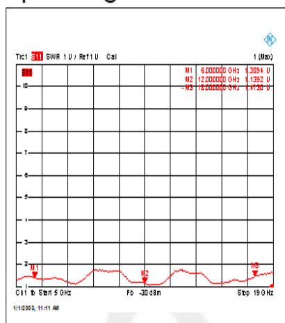
Input VSWR @+25°C
