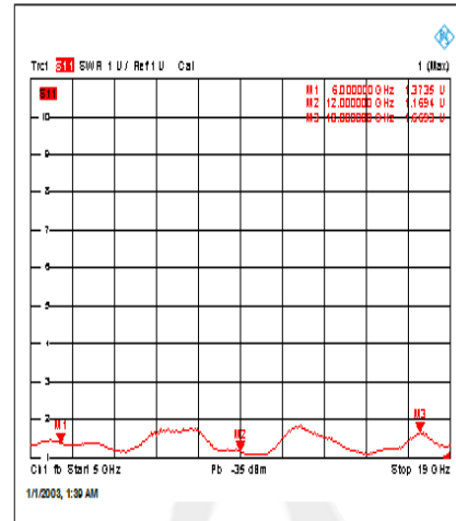
Input VSWR @+85°C
