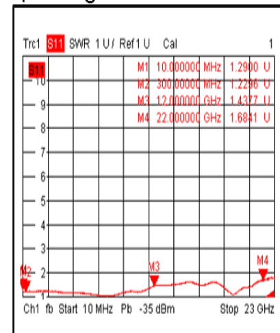
Input VSWR@+85°C
