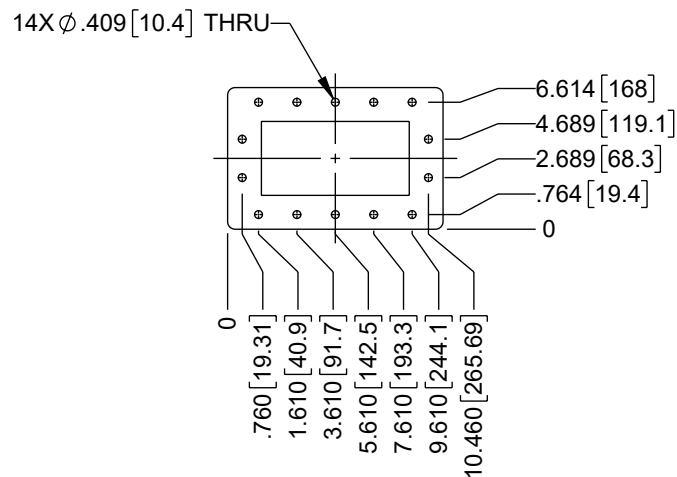
VIEW A-A
